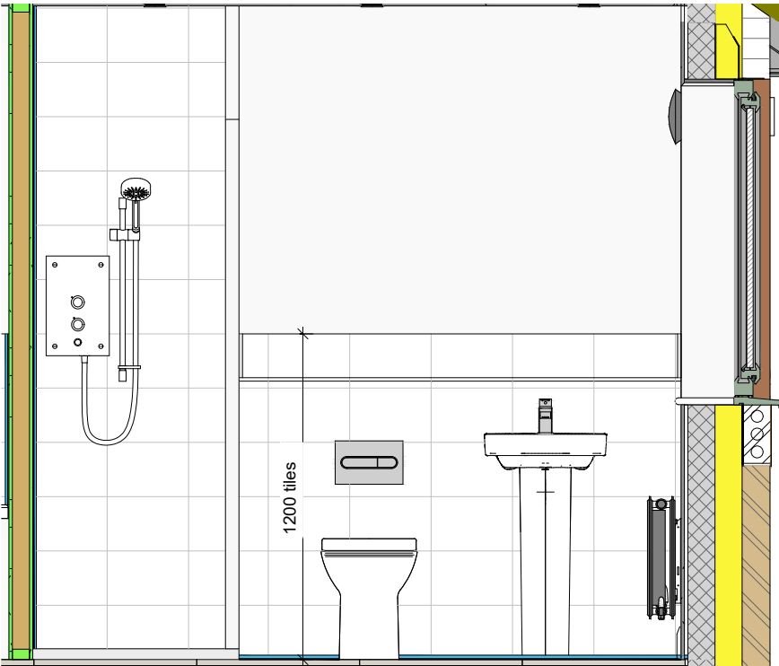
B Ensuite - View B 1 : 25
