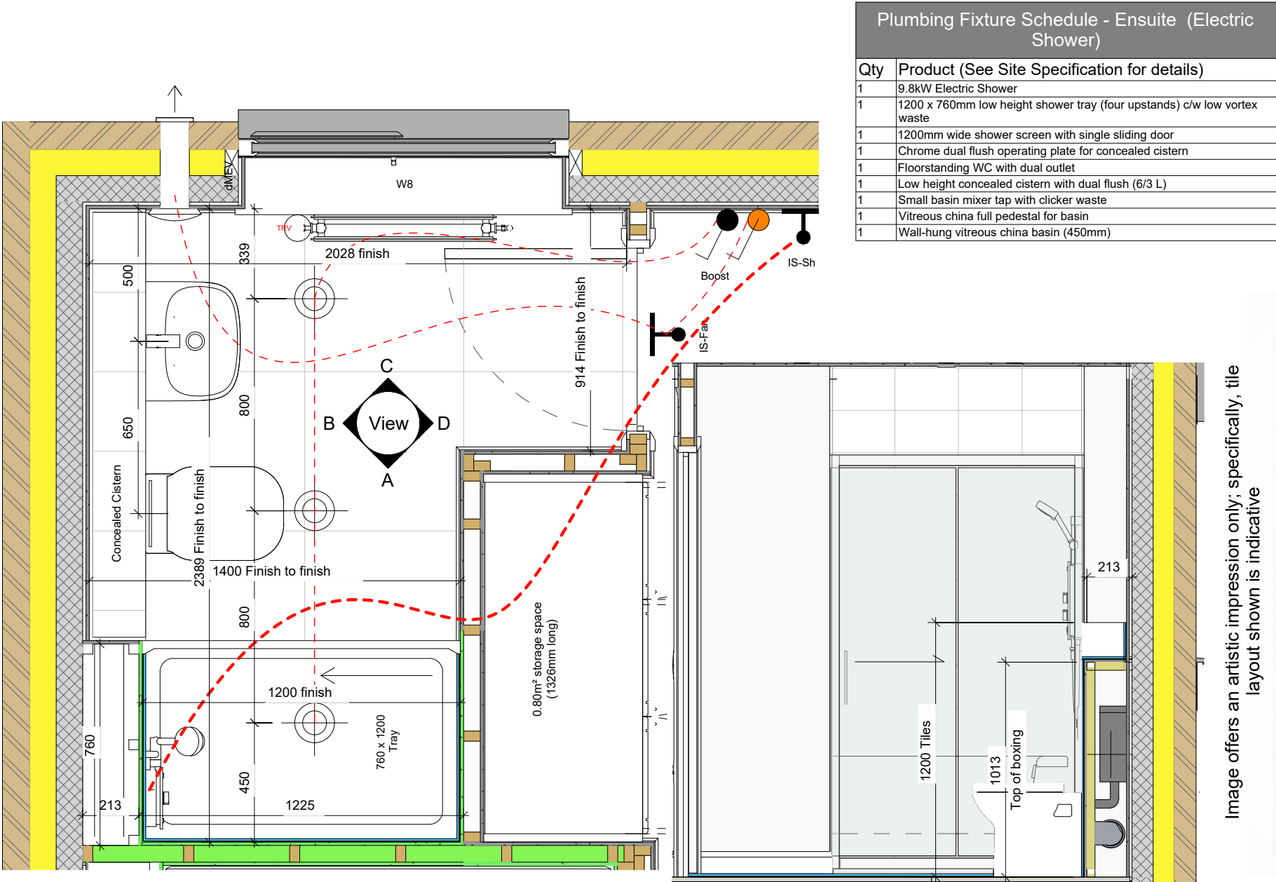
1 Ensuite Layout 1 : 20
