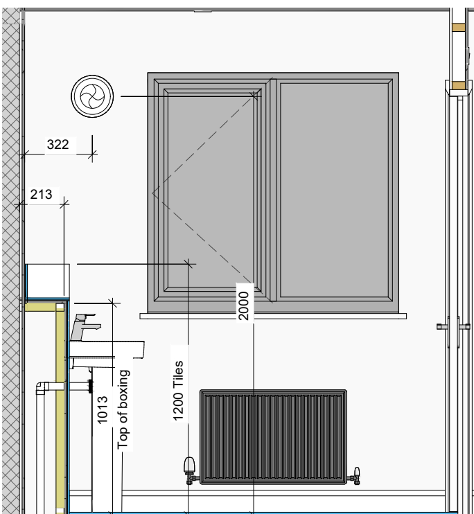
C Ensuite - View C 1 : 25
